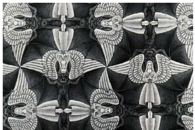
Κανονική διαίρεση του επιπέδου με περιστροφική συμμετρία 90 μοιρών.
