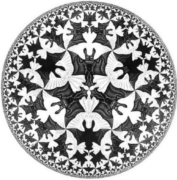
Όριο κύκλου IV Μια οπτική απεικόνιση του κόσμου του Poincaré
