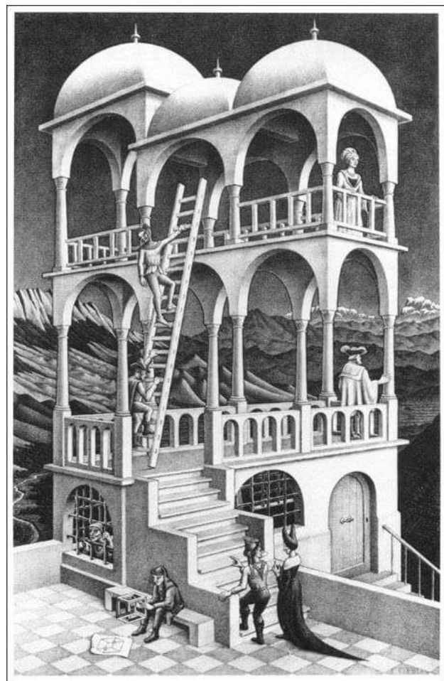
Αδύνατες κατασκευές βασισμένες στην αρχή του στρεβλού τριγώνου.
